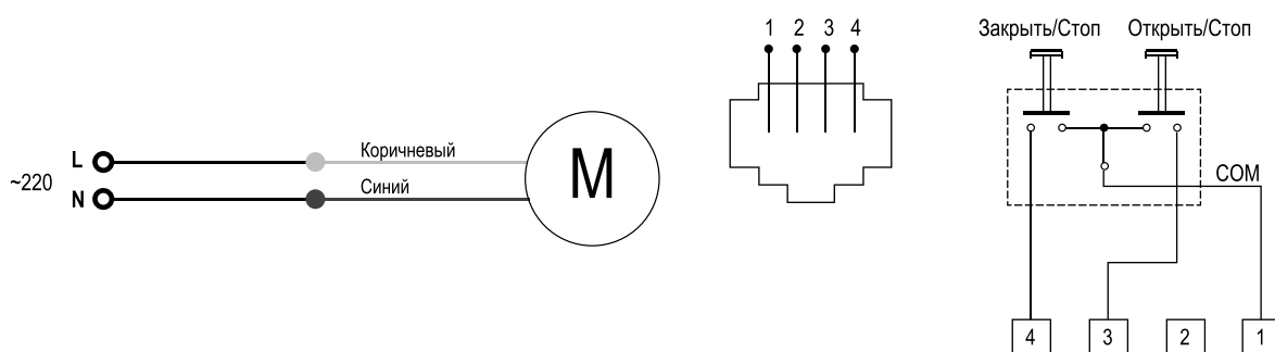
Схема подключения электропривода
